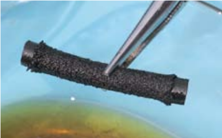
Geschrunpft: Der Textilmantelschlauch hat bei allen Proben gelitten, verwendbar wäre keines der Testexemplare mehr gewesen
